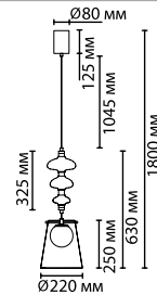
5411/18LB 1 × LED × 18W, 1100 lm крепеж: планка
