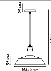
3378/1 1 x E27 x 60W крепёж: планка
