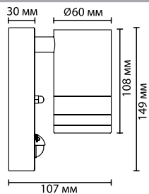
6604/1W, 6605/1W 1 × LED GU10 × 7W крепеж: планка
