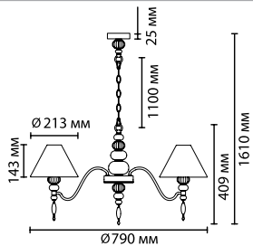
4896/7 7 × E14 × 40W крепёж: планка
