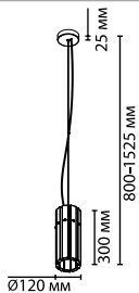
4938/1 1 × E14 × 40W крепёж: планка
