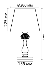
3390/1T, 3393/1T 1 × E14 × 40W выкл. на шнуре
