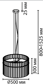
4938/6 6 × E14 × 40W крепёж: планка
