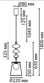
5411/18LA 1 × LED × 18W, 1100 lm крепеж: планка
