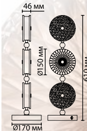
5412/13TL 1 × LED × 13W, 700 lm выкл. на основании
