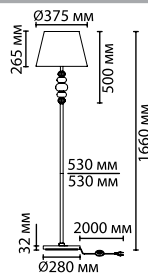
4896/1F 1 × E27 × 60W выкл. на шнуре
