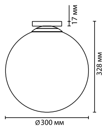
4250/1C 1 × LED E27 × 15W крепеж: планка
