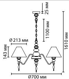
4896/5 5 × E14 × 40W крепёж: планка
