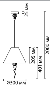
4896/1 1 × E27 × 40W крепёж: планка
