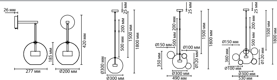
4802/12WL 1 × LED × 12W, 700 Lm крепеж: планка выкл. на базе
