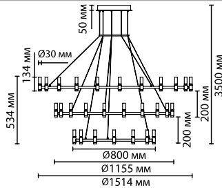
5009/204L 1 × LED × 204W, 4000 lm крепёж: планка
