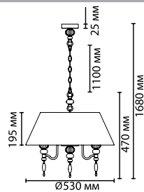
4896/5A 5 × E14 × 40W крепёж: планка
