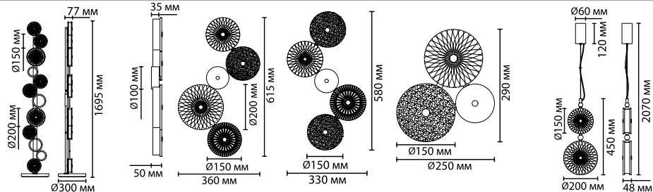
5412/68FL 1 × LED × 68W, 3400 lm выкл. на шнуре 5412/26WL 1 × LED × 26W, 1200 lm крепеж: планка 5412/25WL 1 × LED × 25W, 1100 lm крепеж: планка 5412/14WL 1 × LED × 14W, 600 lm крепеж: планка 5412/13LA, 5412/13LB, 5412/13LC, 5412/13LD 1 × LED × 13W, 700 lm крепеж: планка
