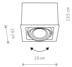
BOX ES111
