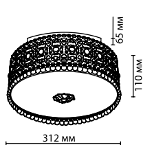
2641/3C 3 x E14 x 40W крепёж: планка
