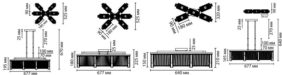
4877/7 7 × E14 × 40W крепеж: планка
