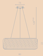
1 7568/02 LM-12 (стр. 19) ∅80 | 122 | 128 mm ⚡ 12x60W E14 Ⓜ 20,6
