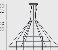
Ø1200+2000+3000+2000+1200 mm E
